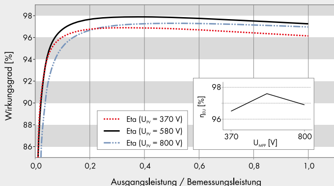
Wirkungsgradkurve SUNNY TRIPOWER 10000TL
